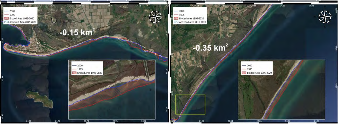
სურათი 2 და 3: კაშხლების ზემოქმედება მდინარე ნესტოსის შესართავების სანაპირო ზონაზე
